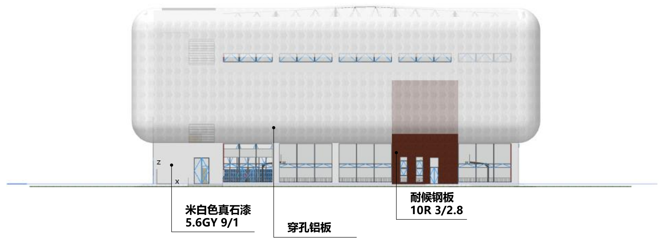
篮球馆2-1轴~2-7轴立面图
