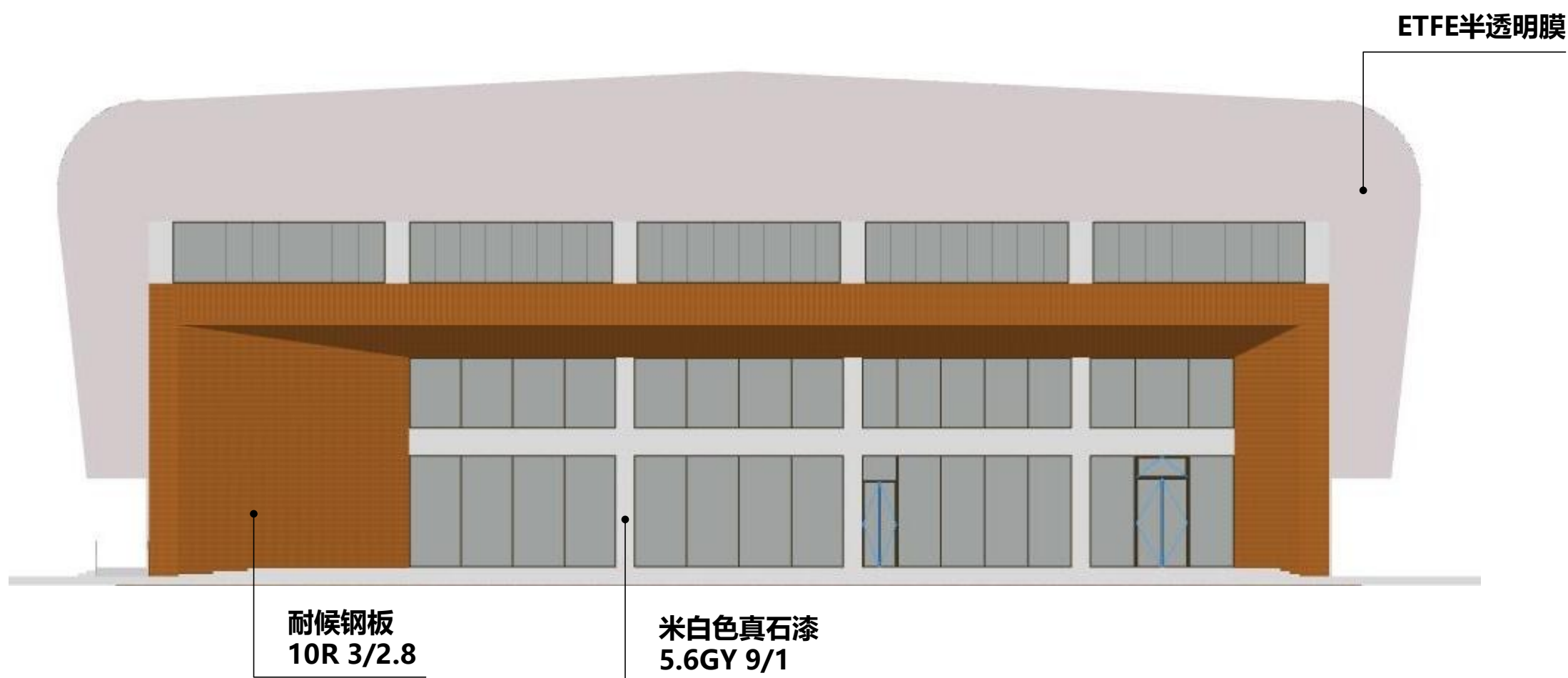
网球馆立面图
