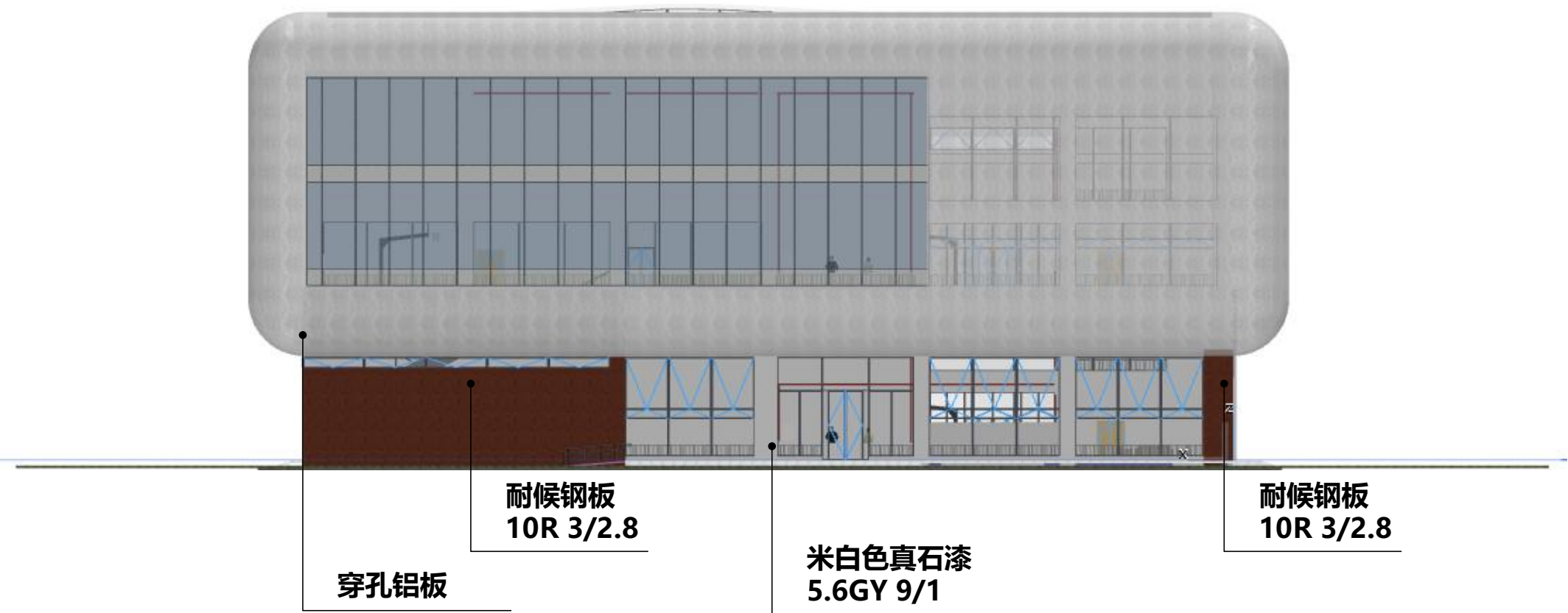
篮球馆2-7轴~2-1轴立面图
