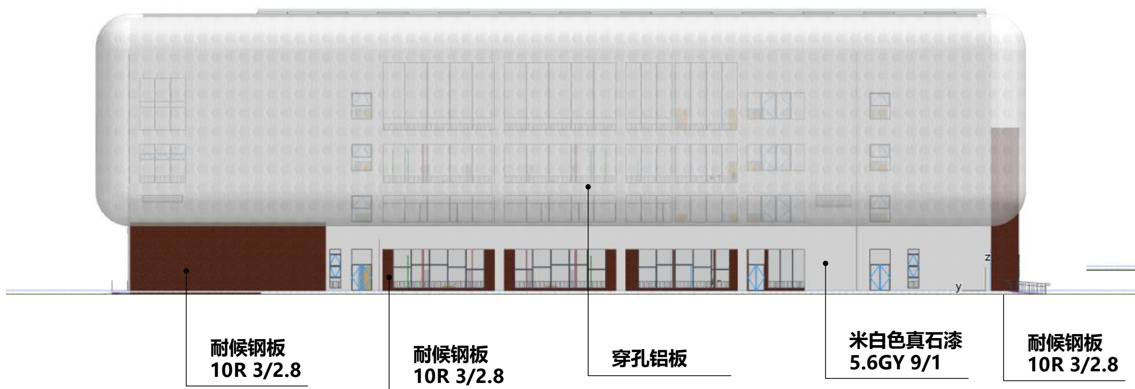
篮球馆2-H轴~2-A轴立面图
