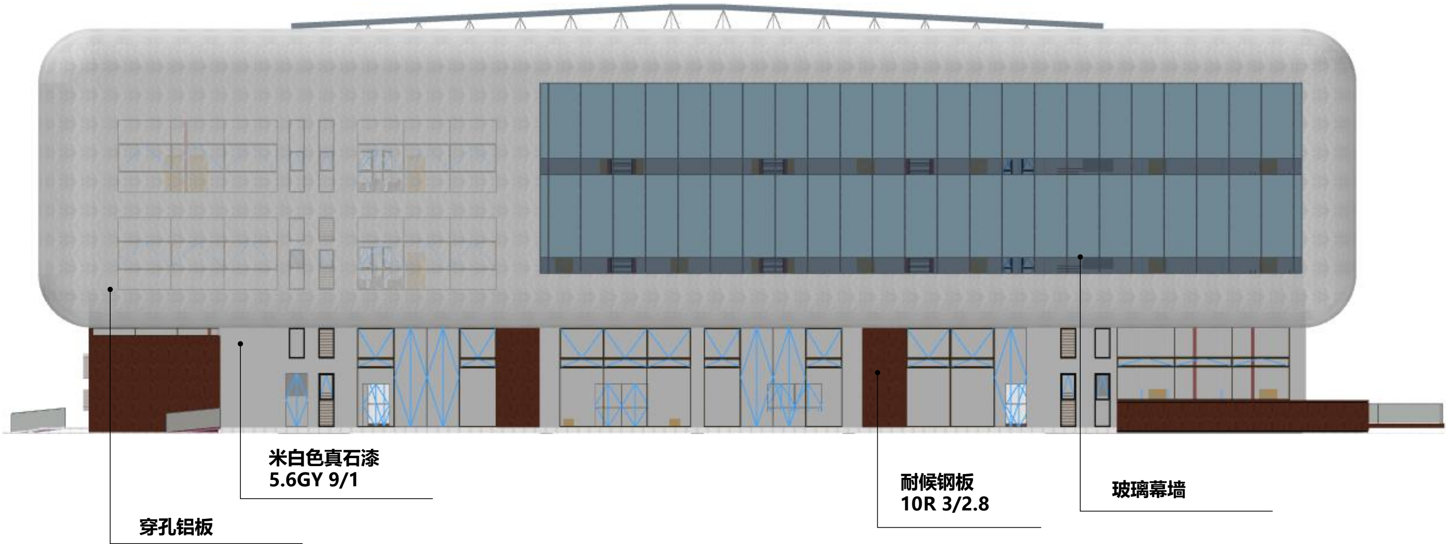
综合馆1-A轴~1-G轴立面图
