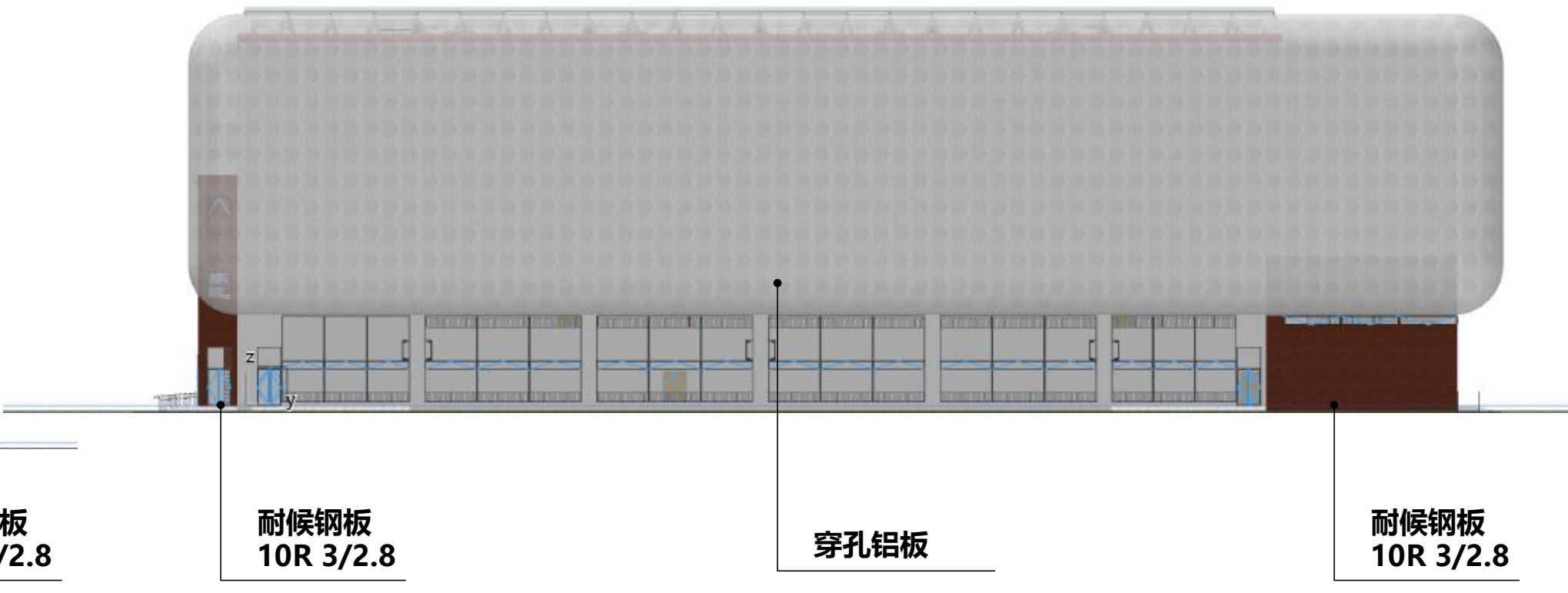
篮球馆2-A轴~2-H轴立面图
